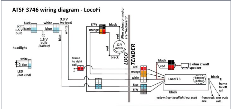
14. LocoFi wiring diagram.
